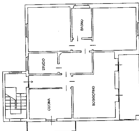
PIANTA PIANO PRIMO H = 3,20
